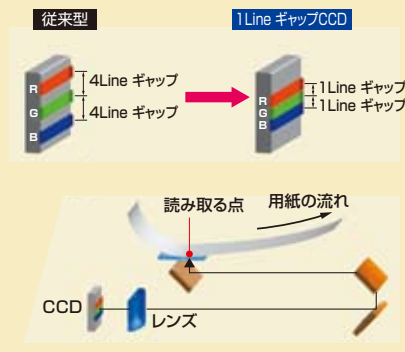
高画質と高生産性を両立する1ラインギャップCCD
